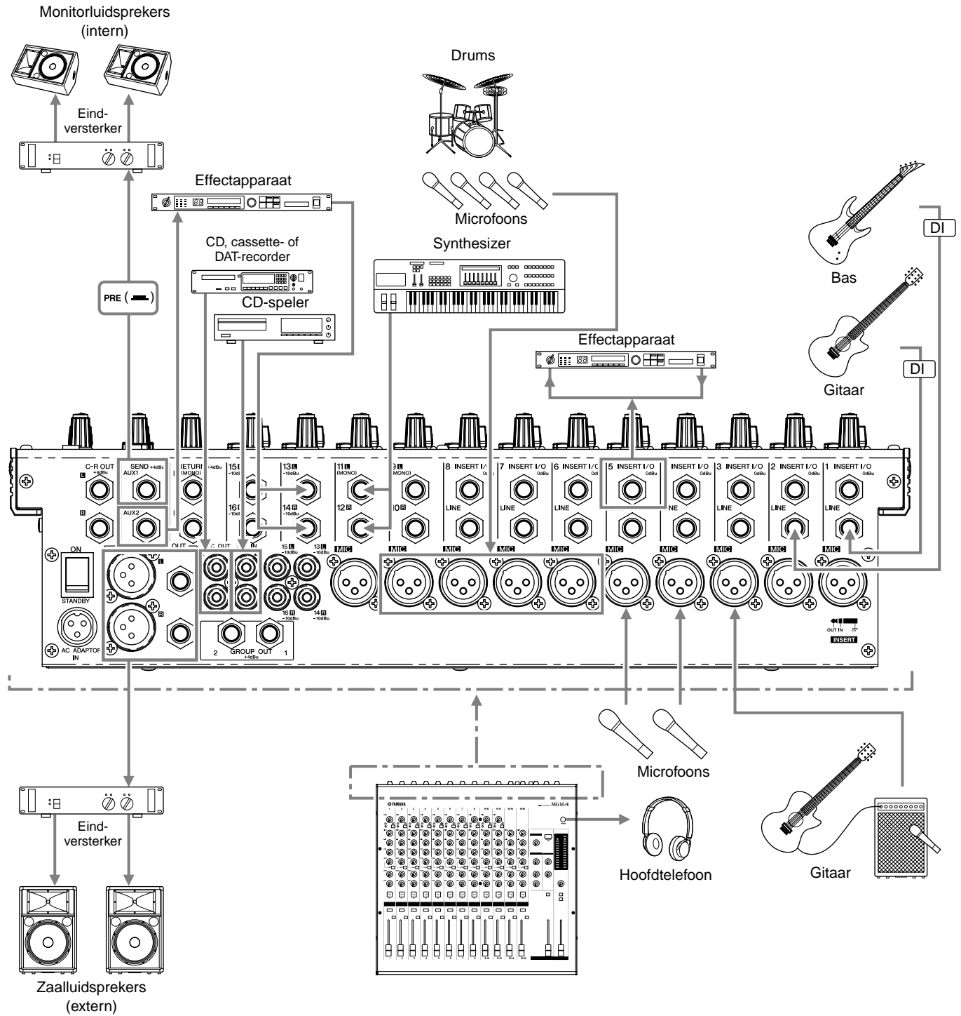
Voorbeeld van een luidsprekeropstelling
