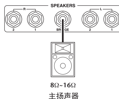
BRIDGE接口上连接
