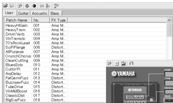
程序库窗口
