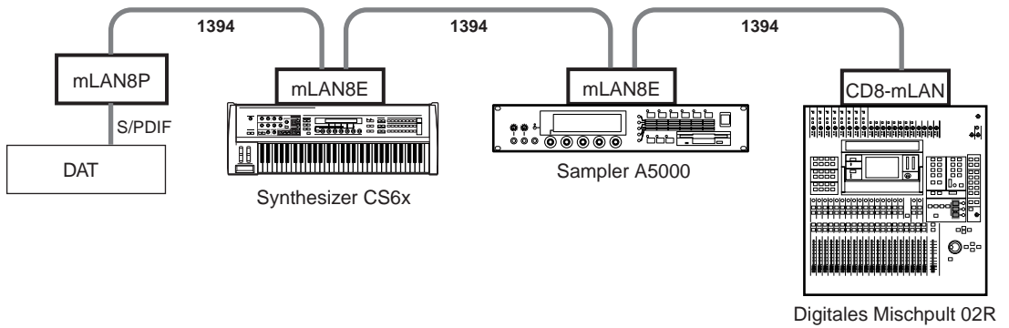
mLAN-Verbindung
