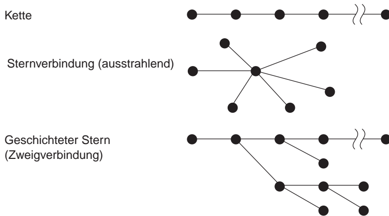
Abbildung 3: Topologiearten
