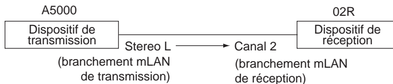
Figure 10 : Un exemple de connexion mLAN
