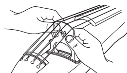
[Le chevalet est placé verticalement]
