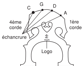
[Echancrure (Vu du cordier)]
