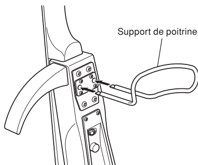
Dos du SILENT Cello™
