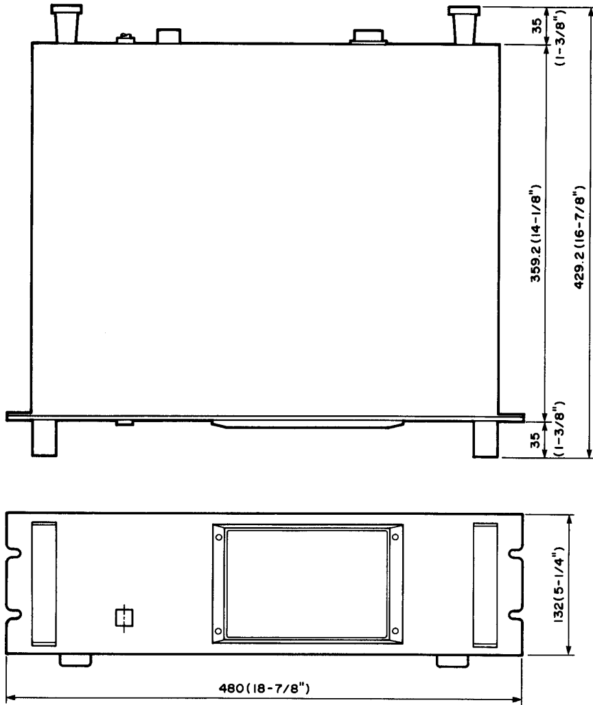
図3-2 PW1800寸法図
