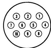
図2-11 PW1800電源供給コネクタピン配列
