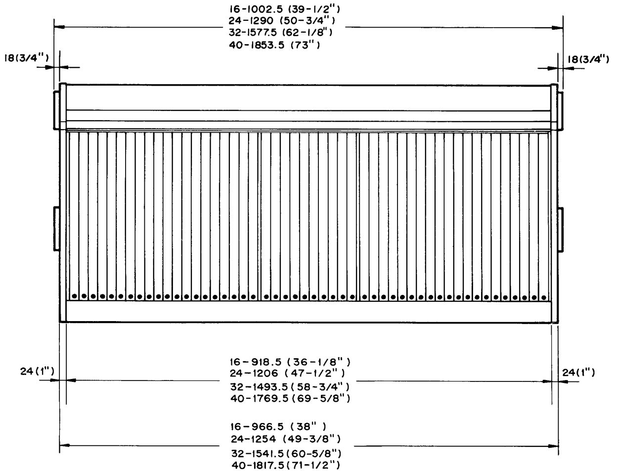
図3-1 PM1800A 寸法図
