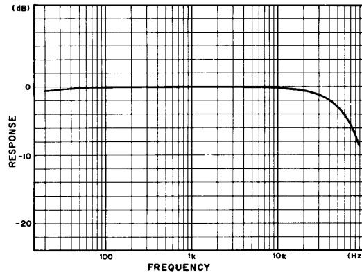
図3-6 周波数特性
