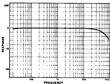
図3-12 周波数特性
