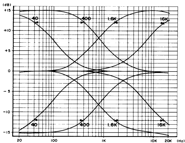
図3-3 HIGHおよびLOW帯域イコライザ特性 (シェルビング)
