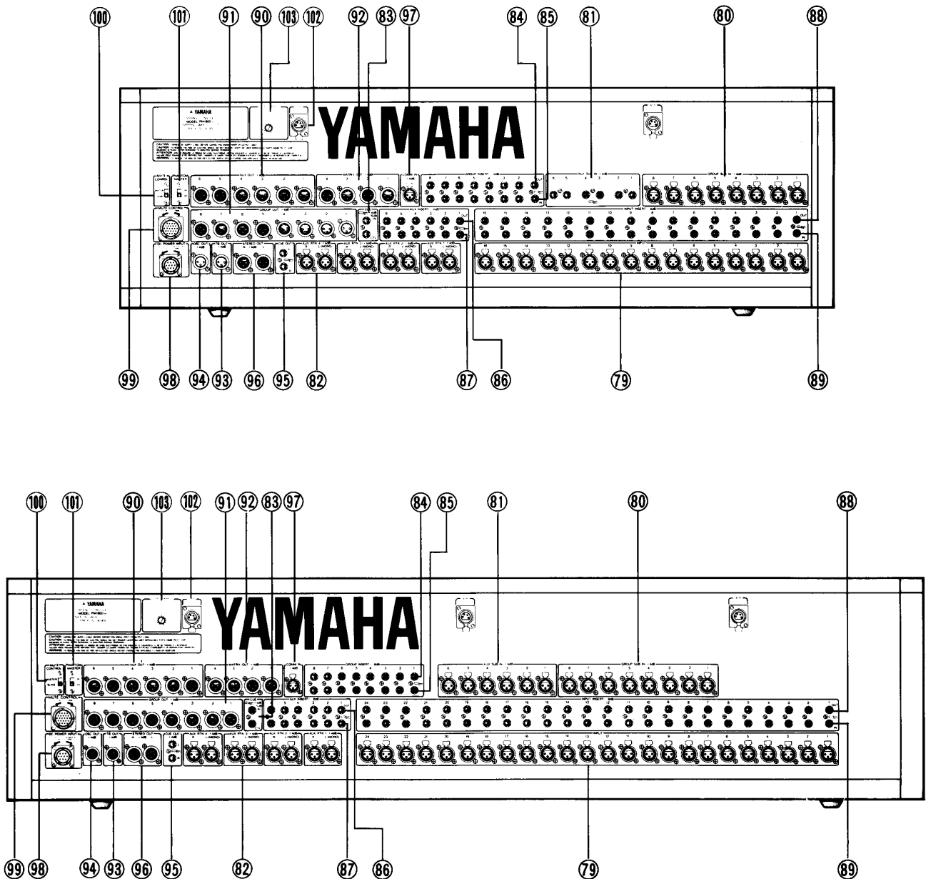
図2-8 PM1800A 後部パネル
