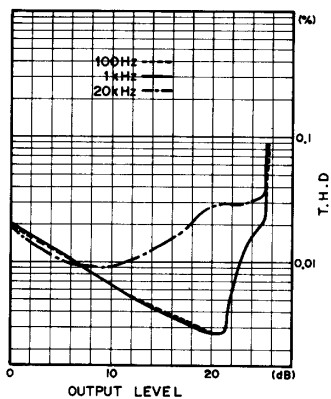
図3-13 出力レベル対全高調波歪
