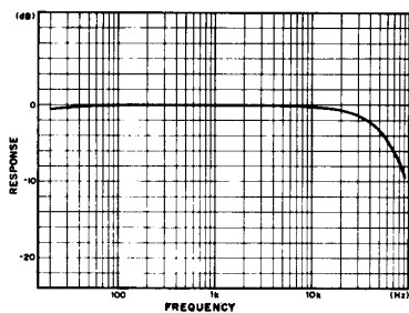
図3-9 周波数特性
