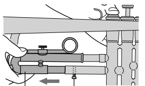
Coulisse de troisième piston Vis d'arrêt de coulisse de troisième piston
